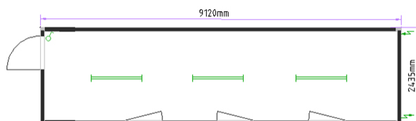
kontener biurowe 30'
