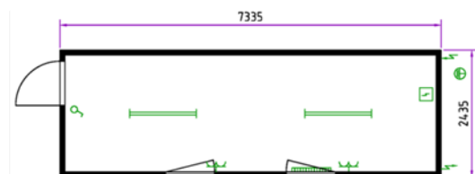
kontener biurowe 24'
