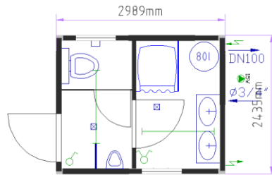
kontener sanitarne 10'
