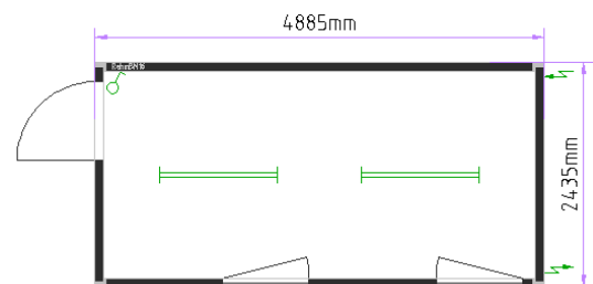
kontener biurowe 16'
