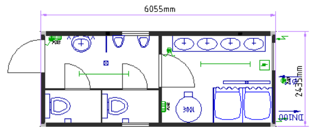
kontener sanitarne 20'
